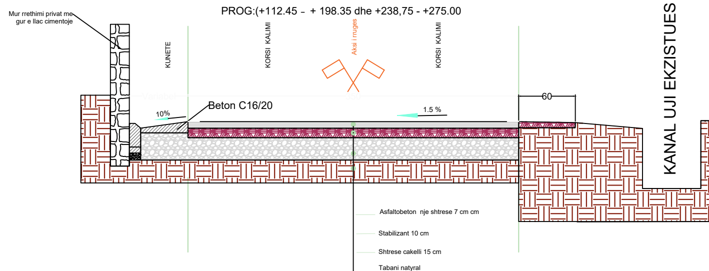
PROFILI TERTHOR TIP 4 ne vendet pa mure ne pjesen jugore dhe ku kanali nuk ngushton trupin e rruges, me kuneten ne krahun e majte SH 1 : 40
