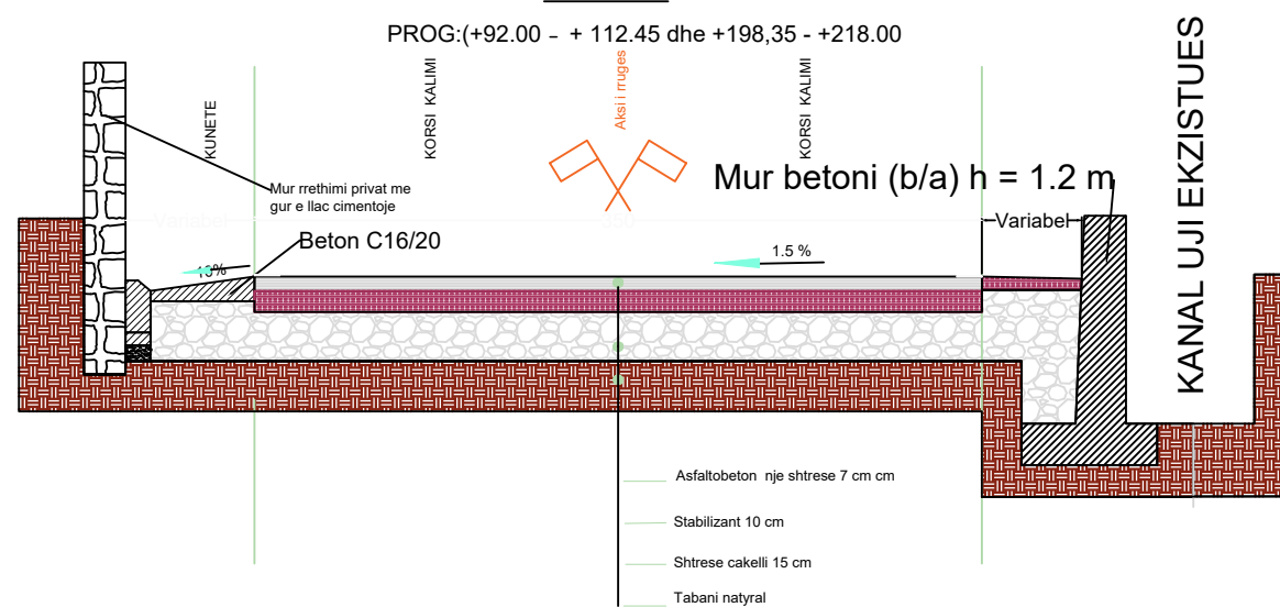
PROFILI TERTHOR TIP 2 SH 1 : 40
