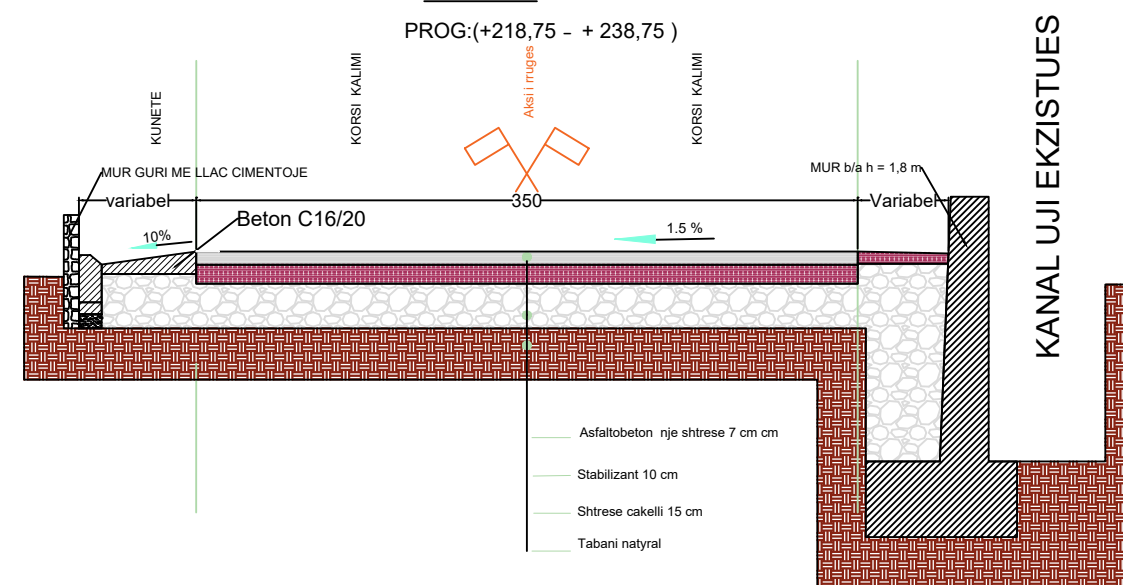
PROFILI TERTHOR TIP 2' SH 1 : 40
