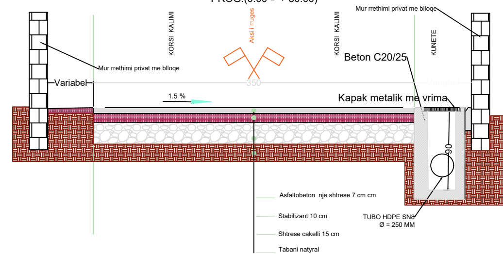
PROFILI TERTHOR TIP 1' PRERJE NE AKSIN E PUSETES
