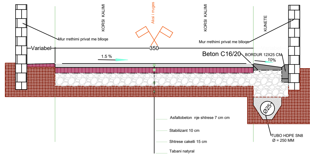
PROFILI TERTHOR TIP 1 SH 1 : 40
