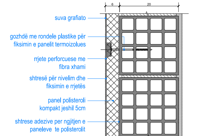
6 DETAJ I VESHJES A CAPPOTTO 1:10
