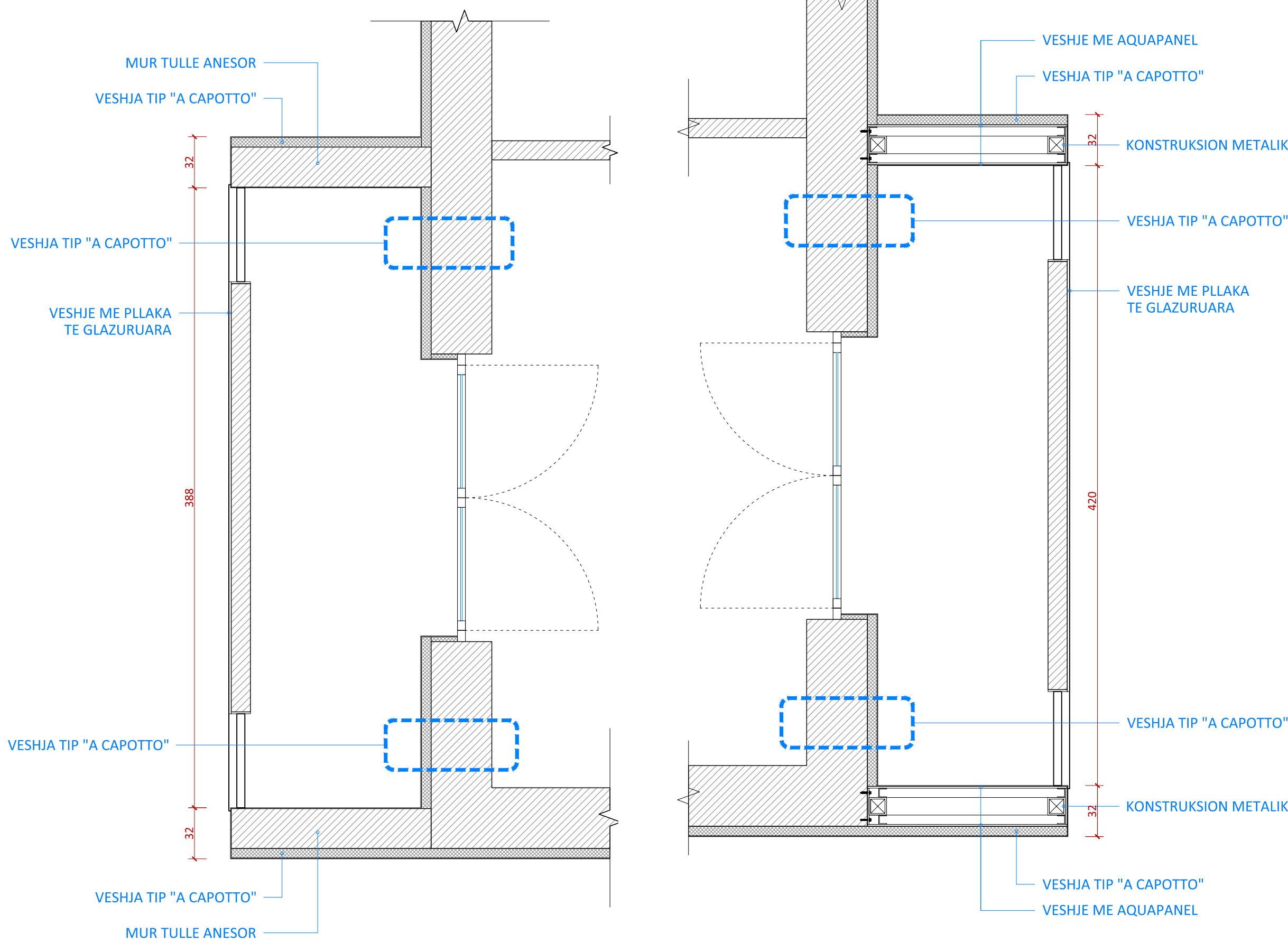
3 DETAJ I BALLKONEVE EKZISTUESE 1:25
