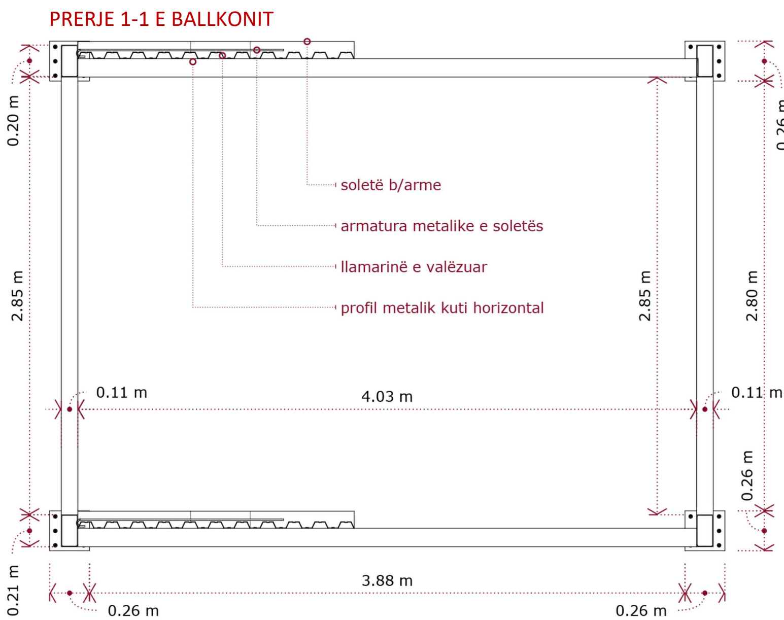
2 DETAJ I BALLKONEVE QE SHTOHEN 1:25
