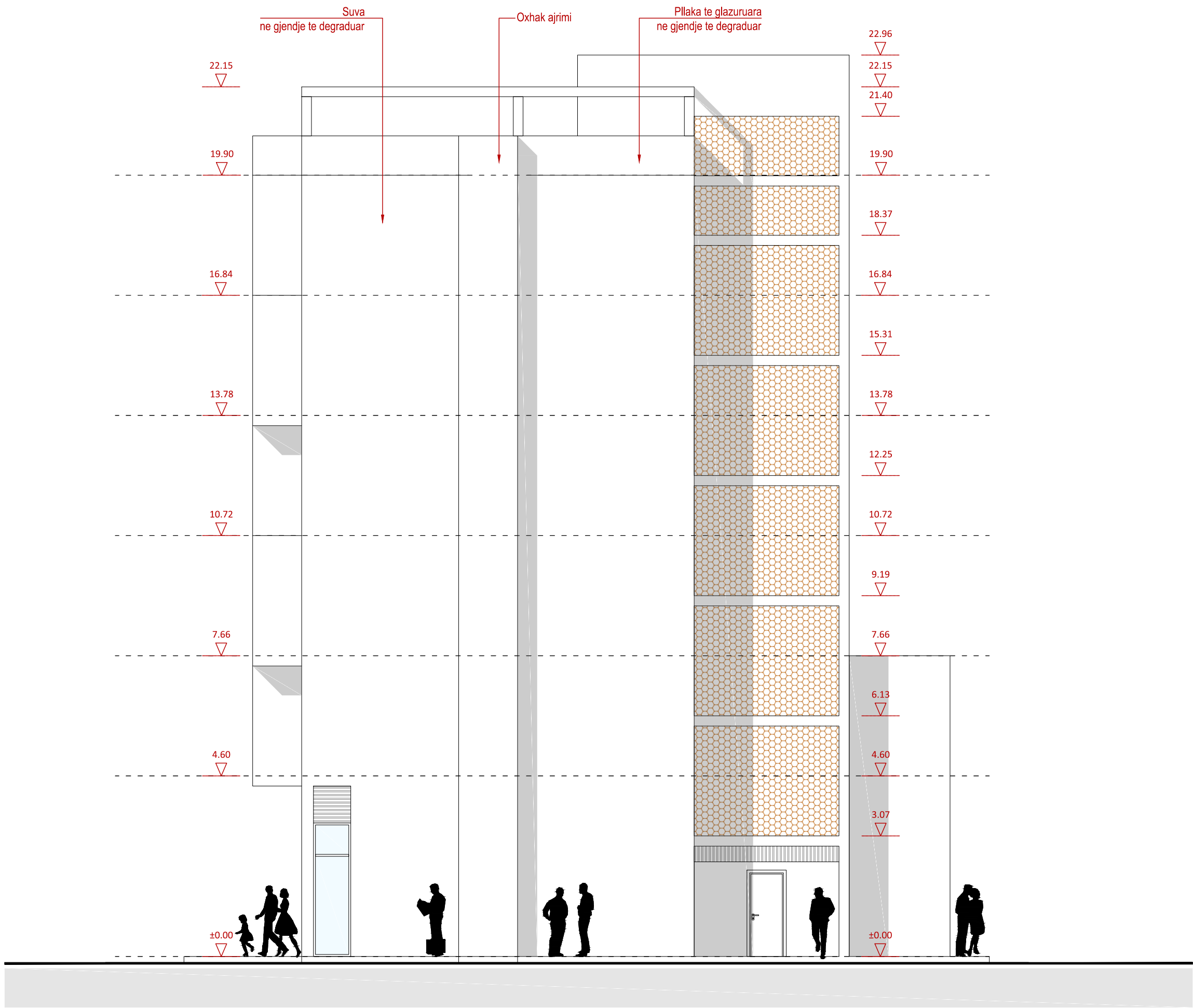
1 PAMJE NGA VERILINDJA 1:100
