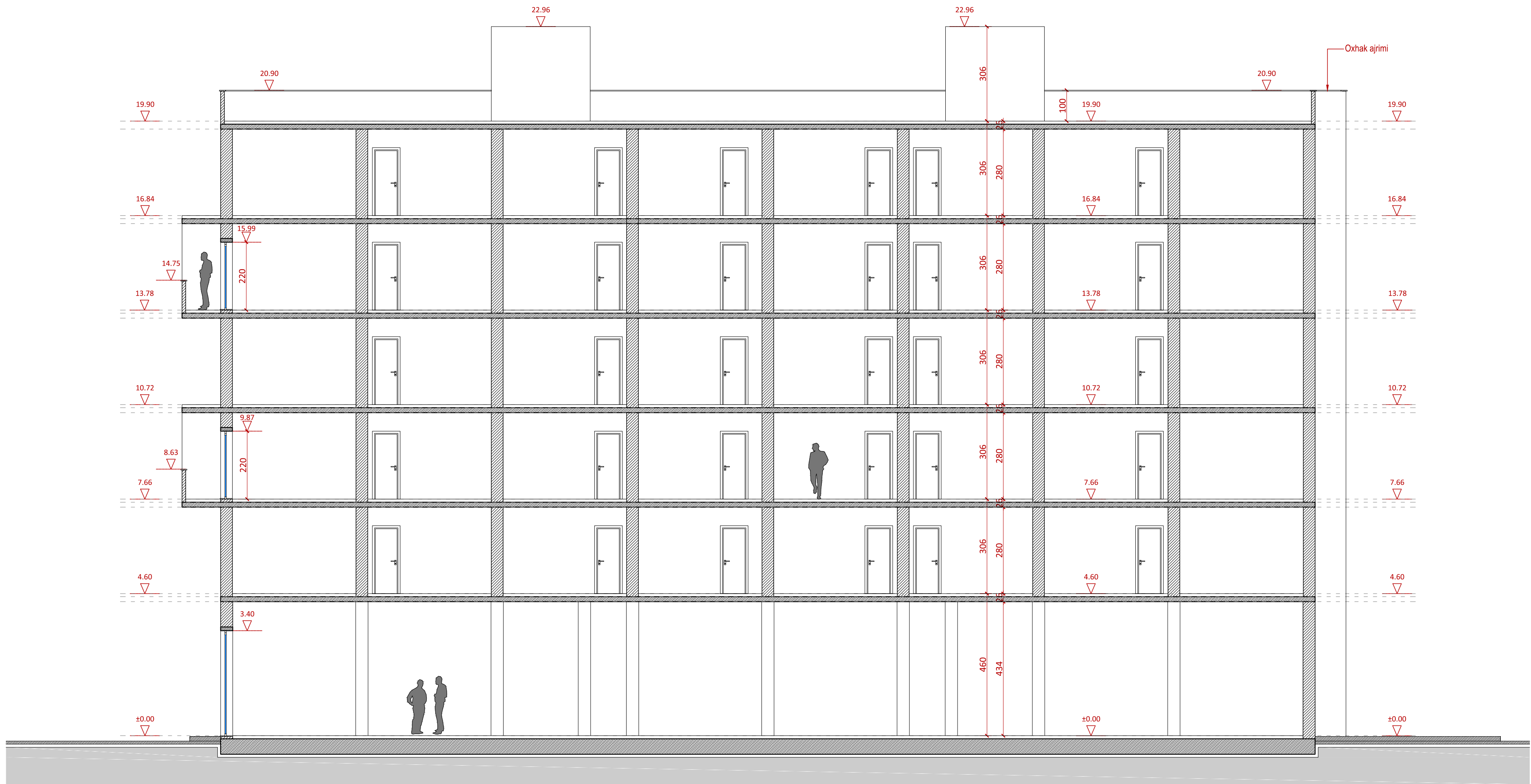
1 PRERJE 1-1 1:100
