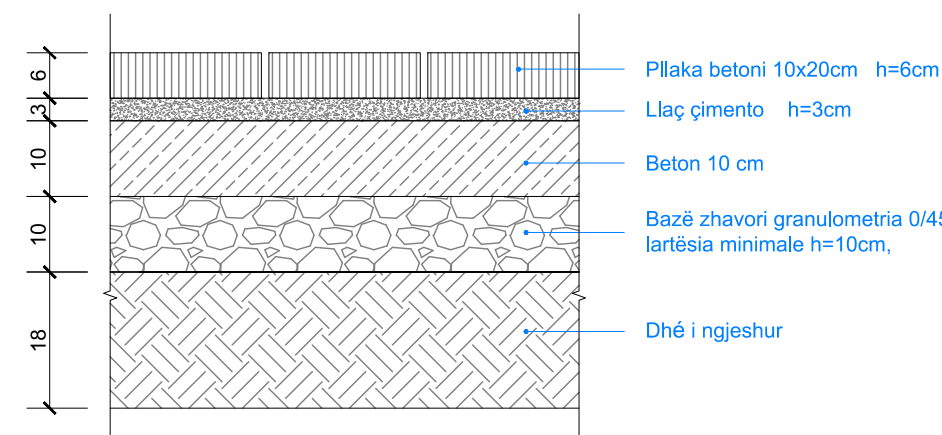
7 DETAJ I SHITESAVE TE TROTUARIT 1:10
