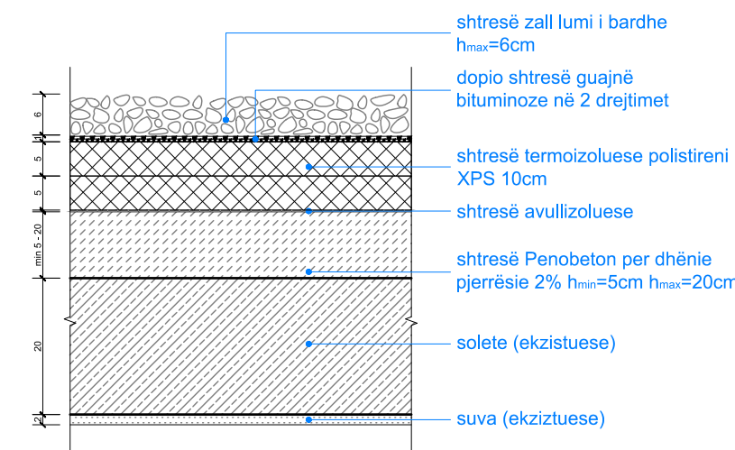
5 DETAJ I SHITESAVE NE TARACE 1:10
