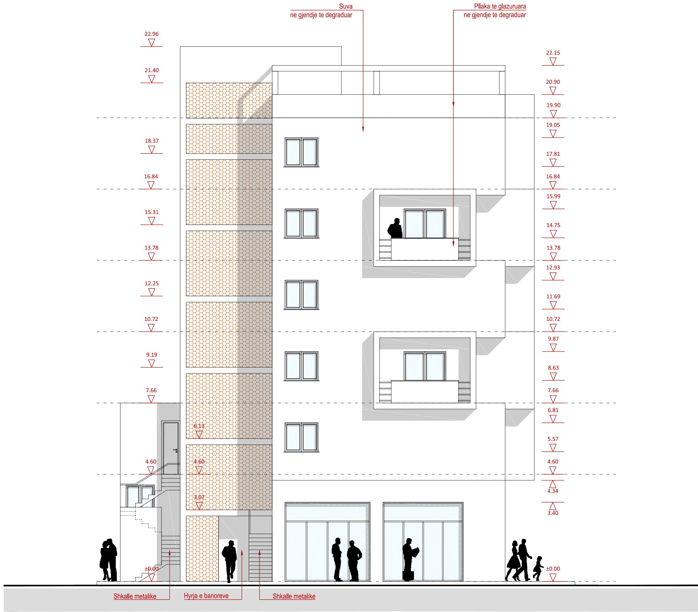
2 PAMJE NGA JUGPERËNDIMI 1:100
