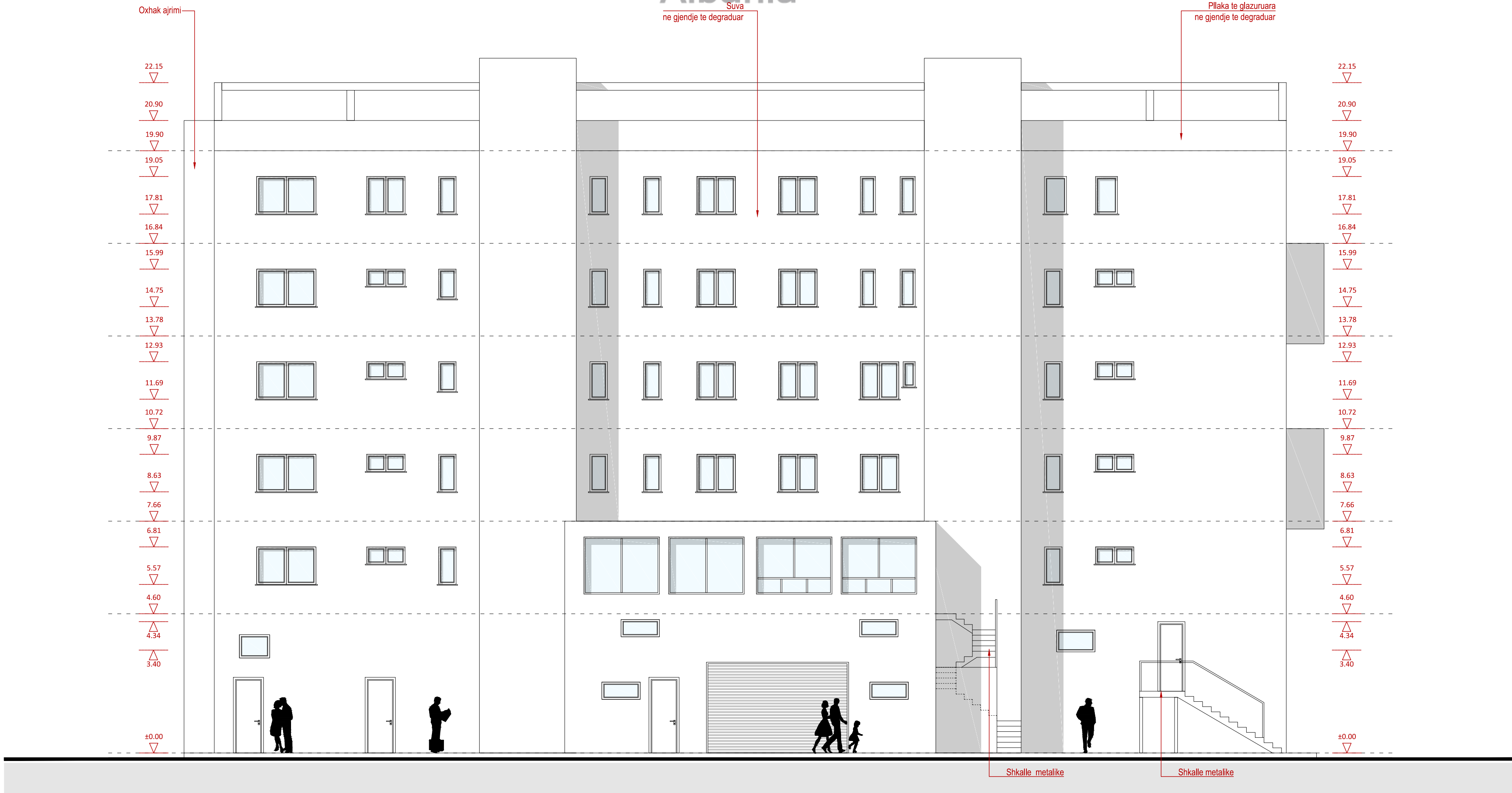
2 PAMJE NGA JUGPERËNDIMI 1:100
