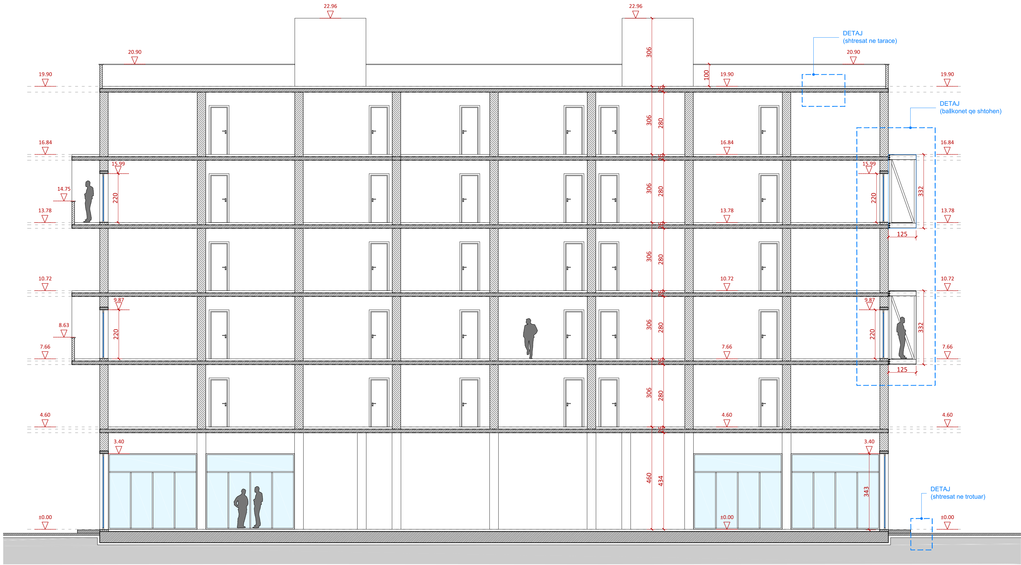
1 PRERJE 1-1 1:100 PLANIMETRI E BALLKONIT
