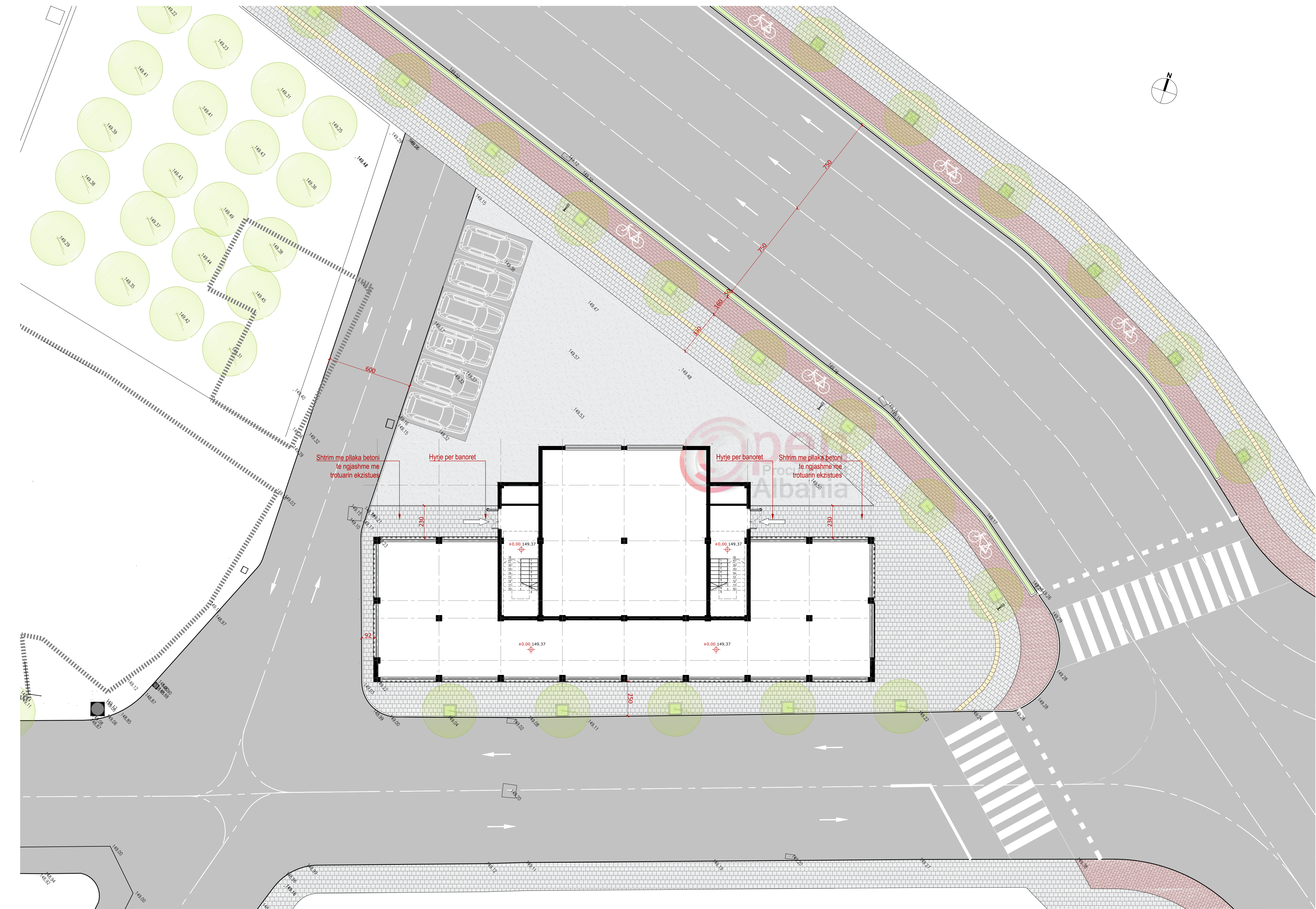
1 PLANI I SISTEMIMEVE 1:150
