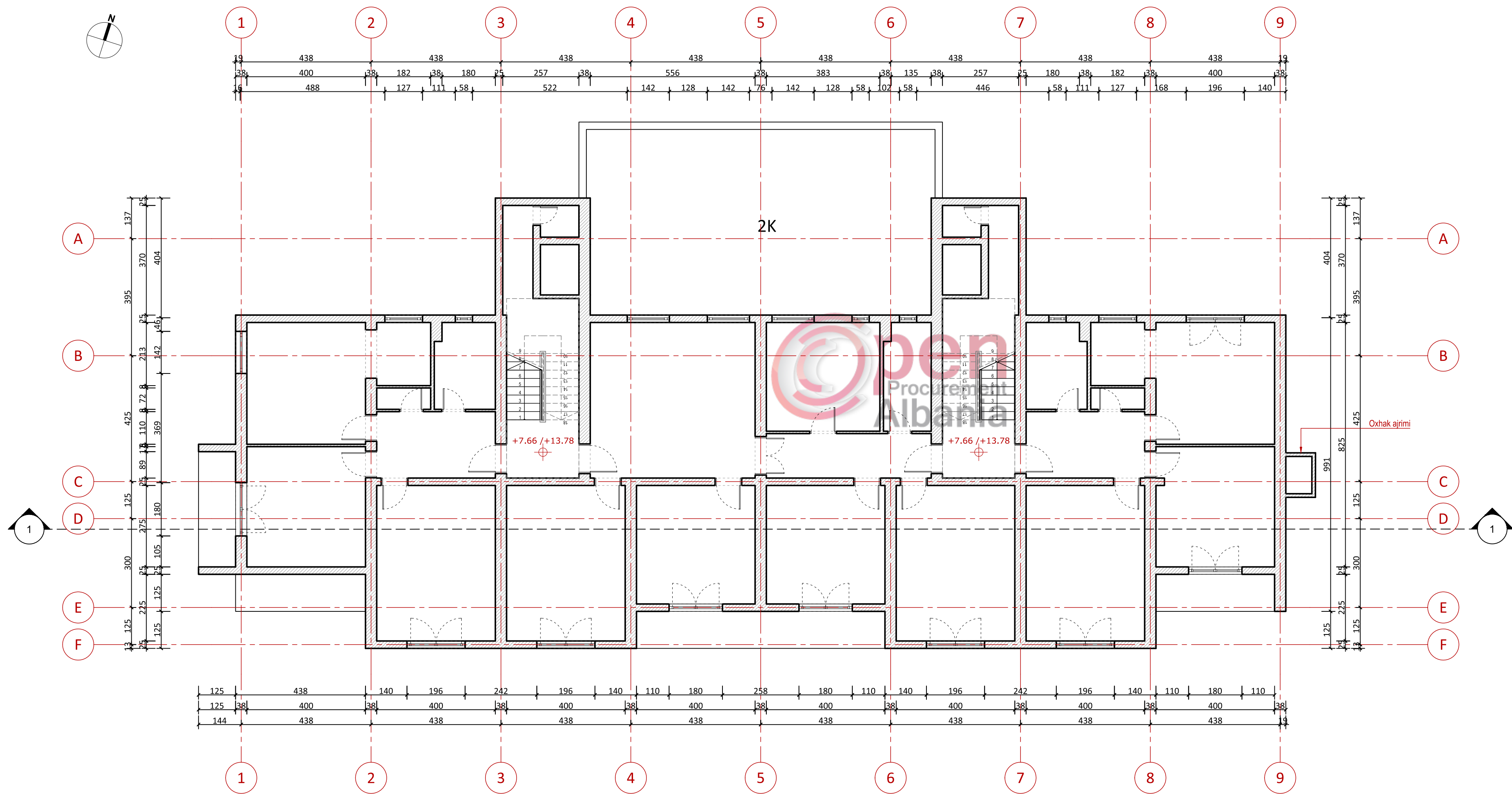
1 PLANIMETRIA E KATIT TË DYTË DHE TË KATËRT 1:100
