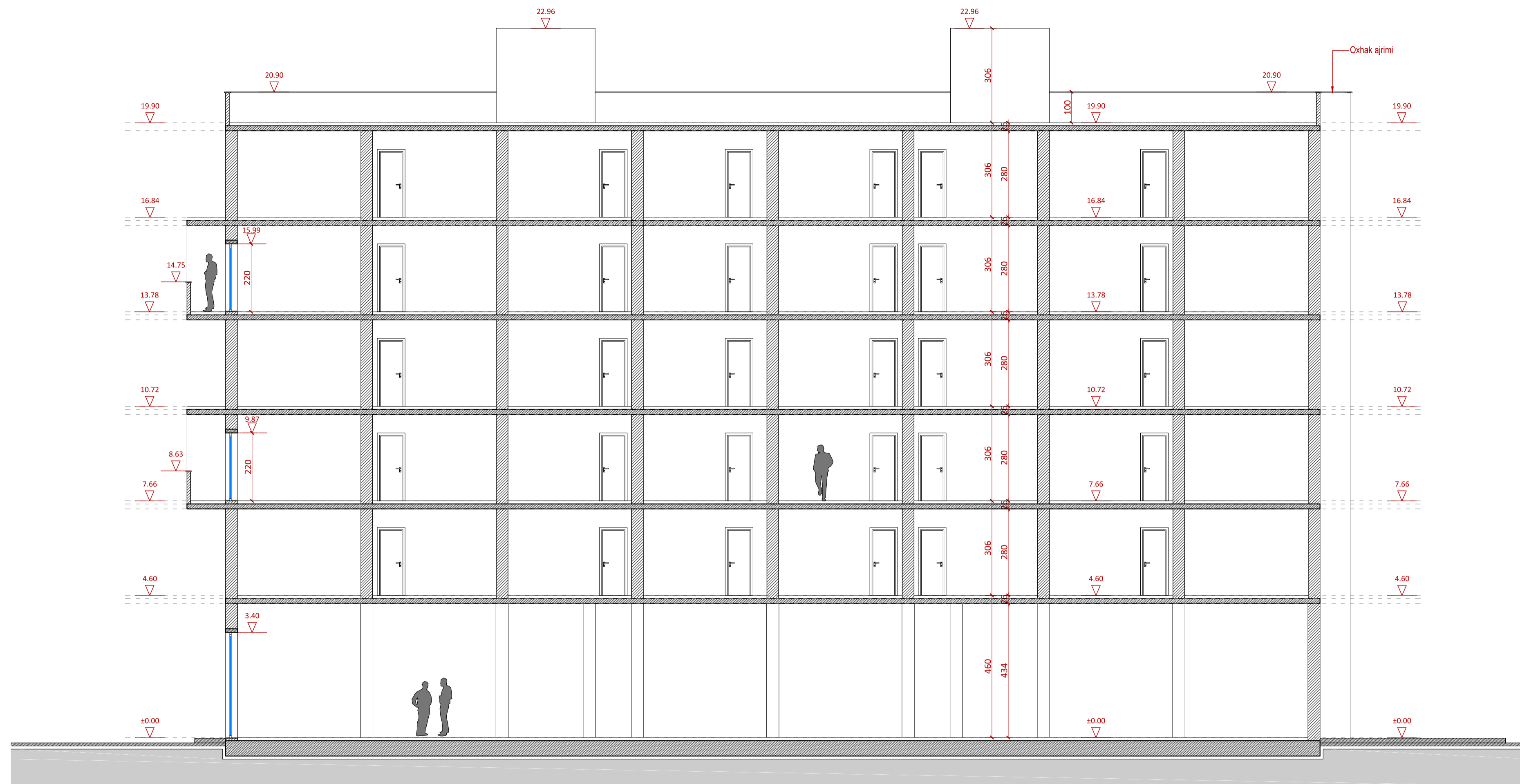
1 PRERJE 1-1 1:100
