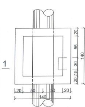
PLANIMETRIA
