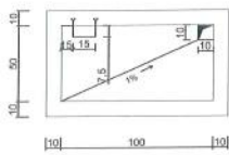
MBULIMI I PUSETES SHK.1:50
