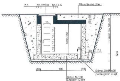
PRERJA 1-1 SHK.1:50
