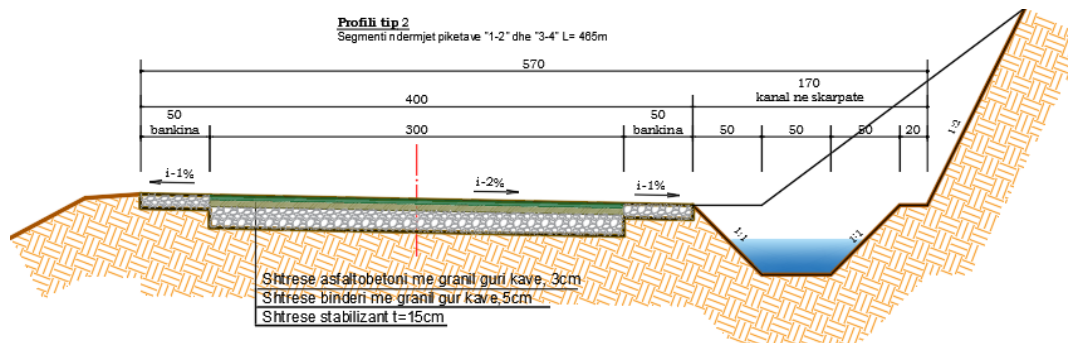
Fig. 3 Profili tërthor "Tipi 2"
