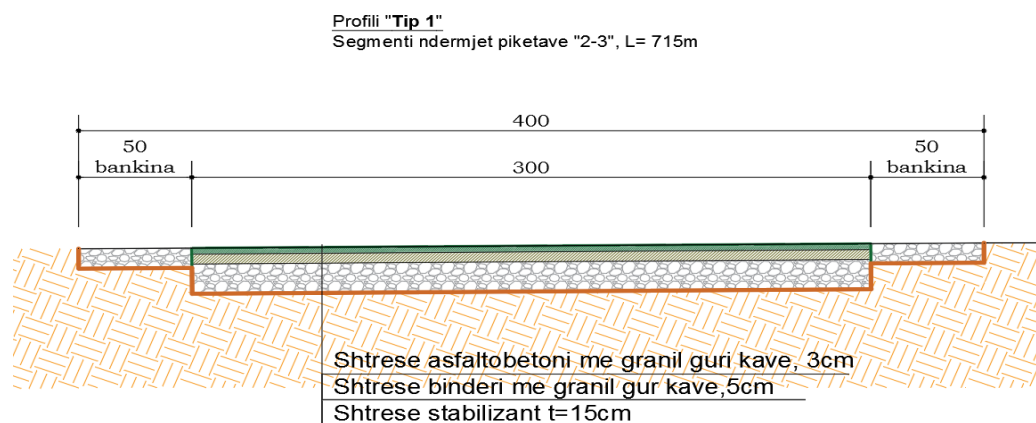
Fig. 2 Profili tërthor "Tipi 1"
