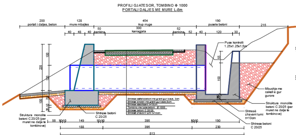
Fig. 4 Prekje gjatësore e tombinos Φ1000.
