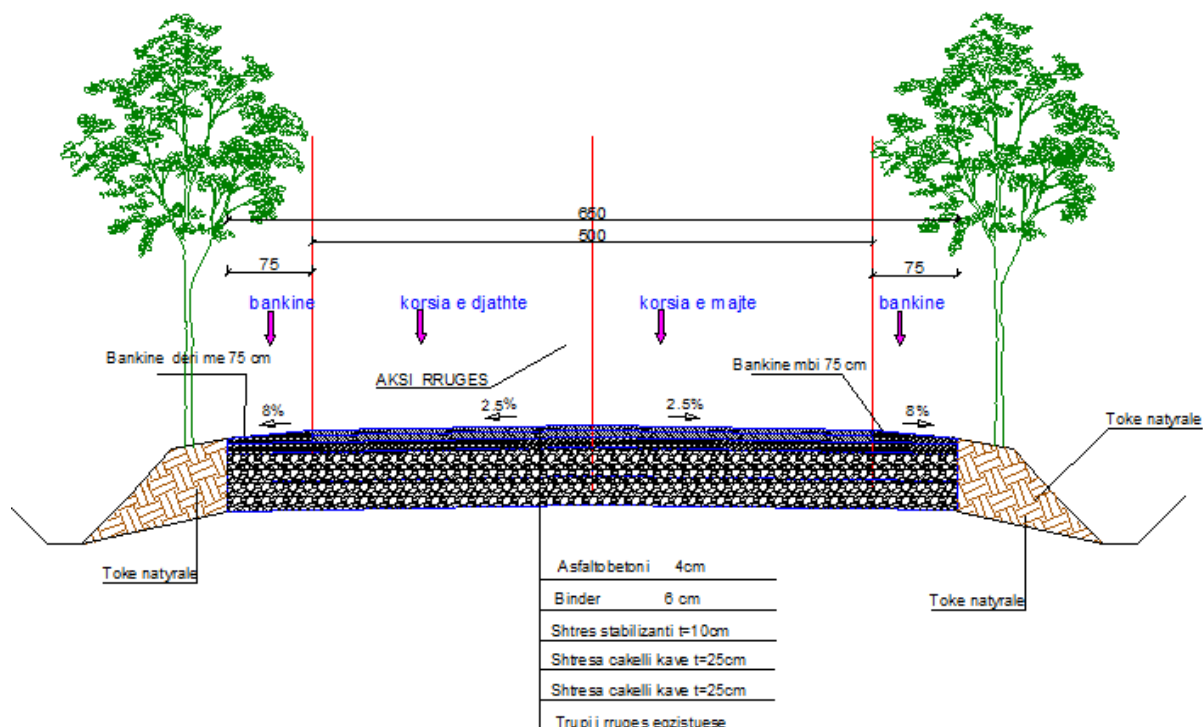
Fig.7 Profil tip
