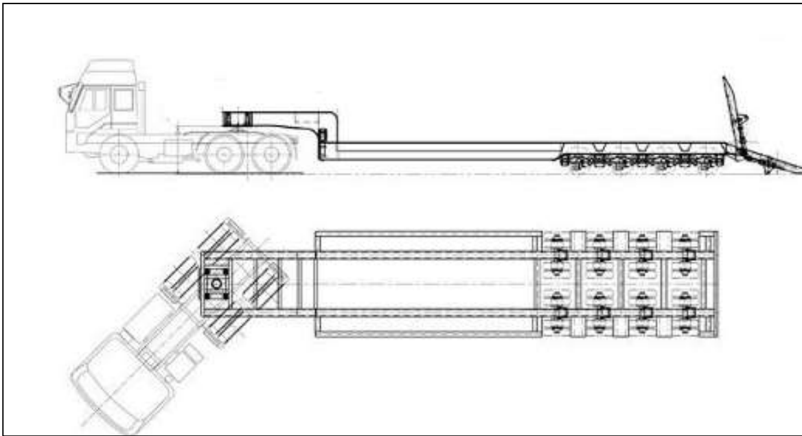
Skema teknike Tërheqës plus Gjysëmrorkio;
