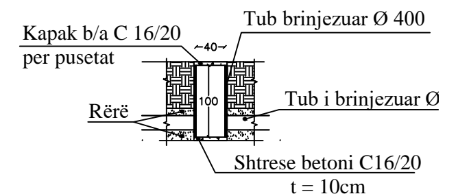
PRERJA A-A E PUSETE SHKARKIMI
