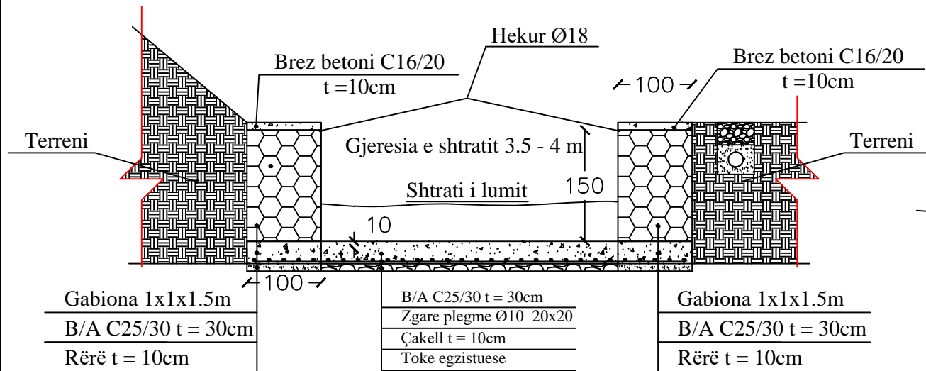
PRERJA TERTHORE TIP E LUMIT
