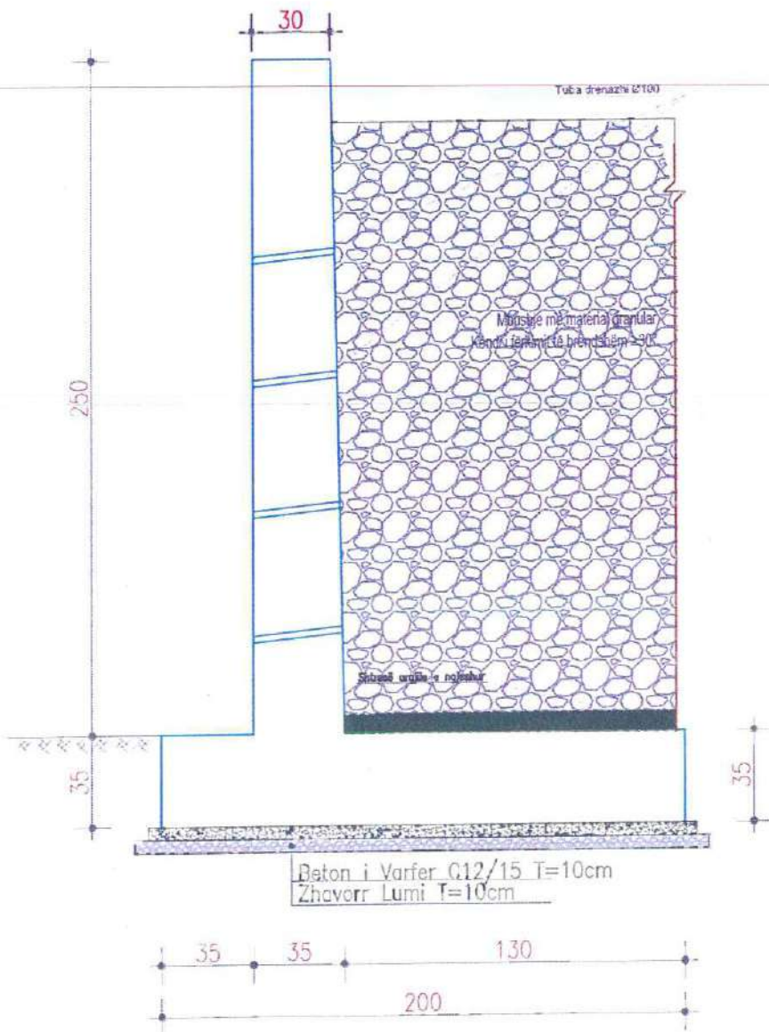
MURI MBAJTËS B/A H=2.5m, L=1.0m
