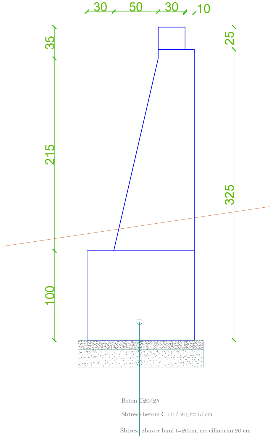
PROFILI TIP MURI MBAJTES
