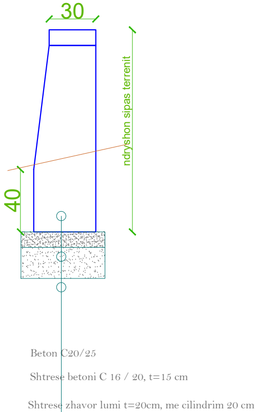
PROFILI TIP MURI RAKORDUES ME TERRENIN
