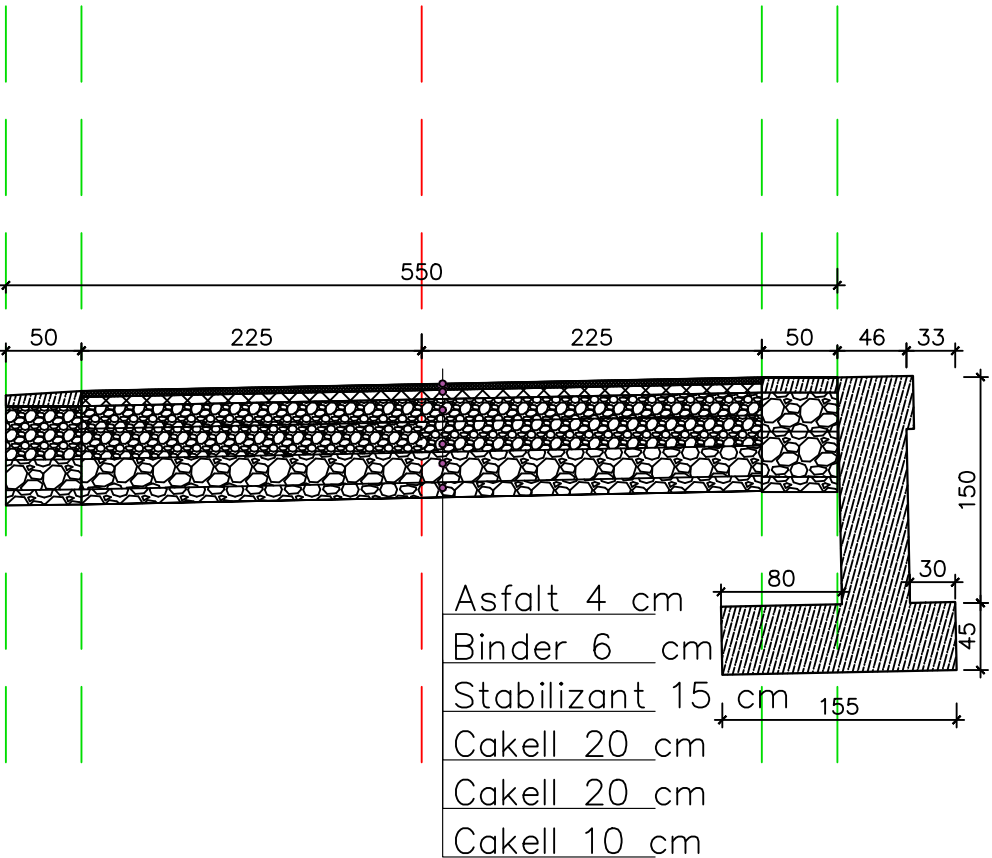
PROFIL TIP 2 Prog0+604.00 -0+660.00
