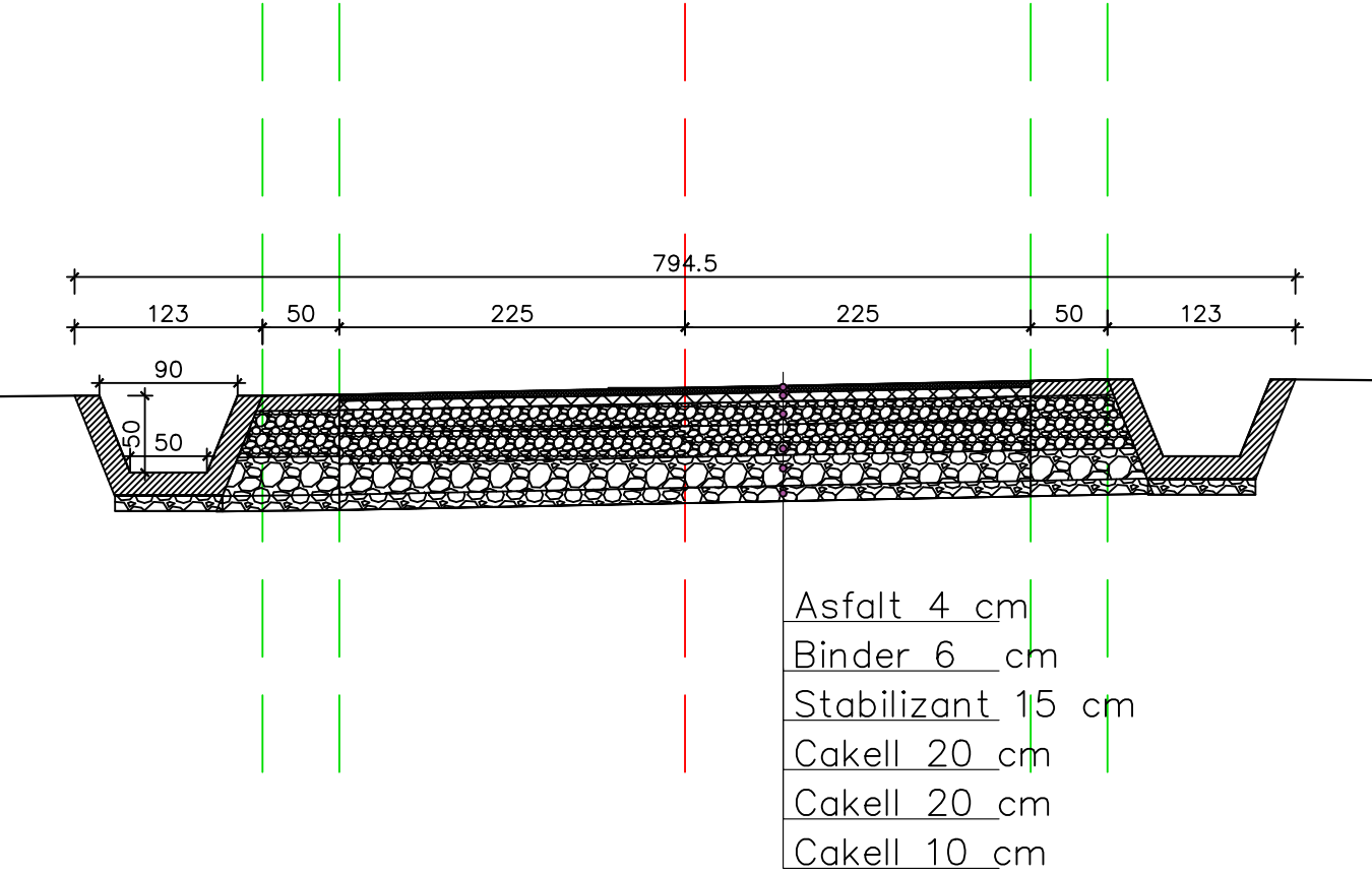
PROFIL TIP 2 Prog0+604.00 -0+660.00
