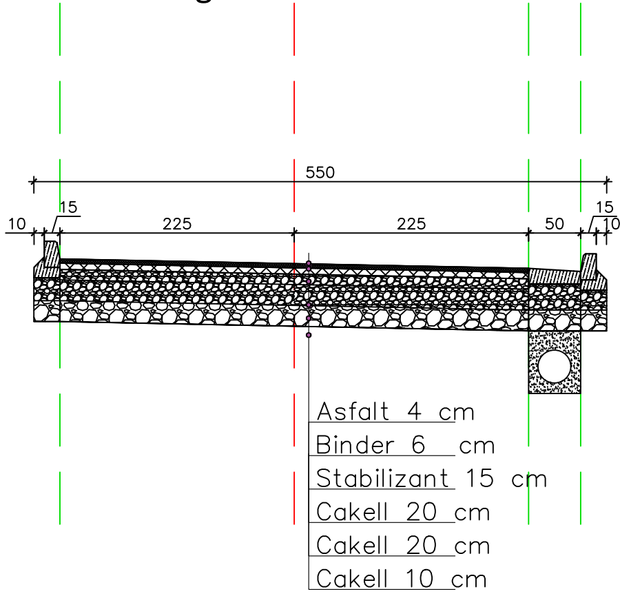
PROFIL TIP 1 Prog0+000.00-0+45.00
