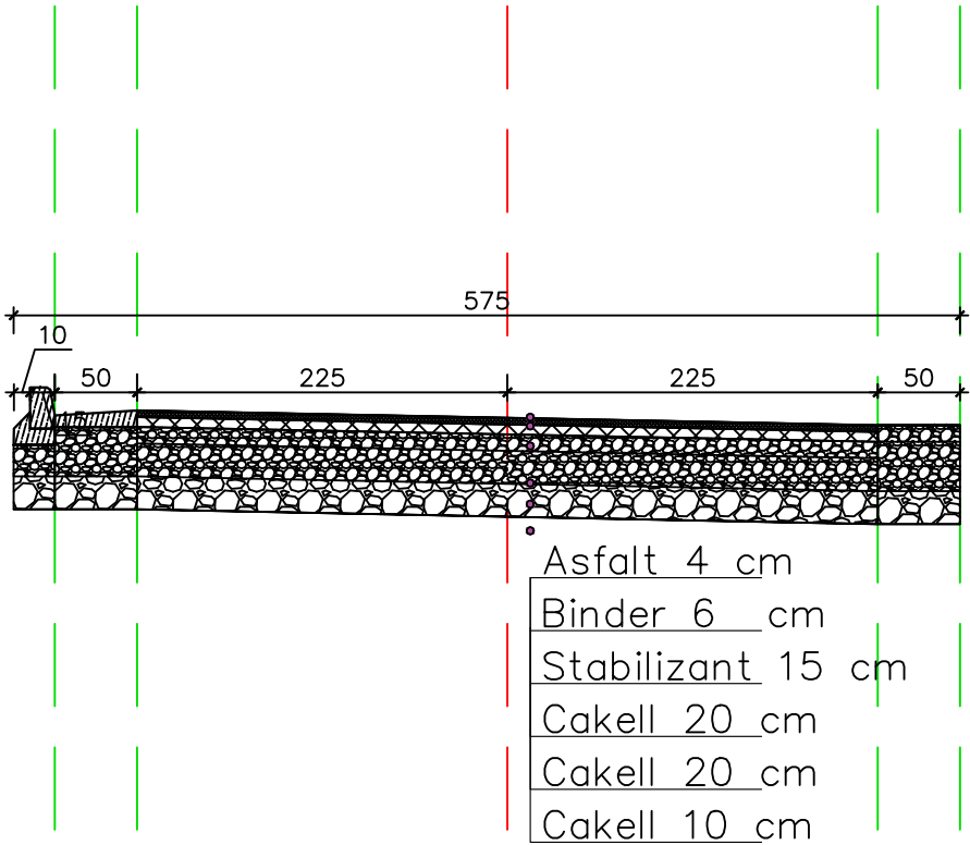
PROFIL TIP 4 Prog0+822.00 -1+000.00
