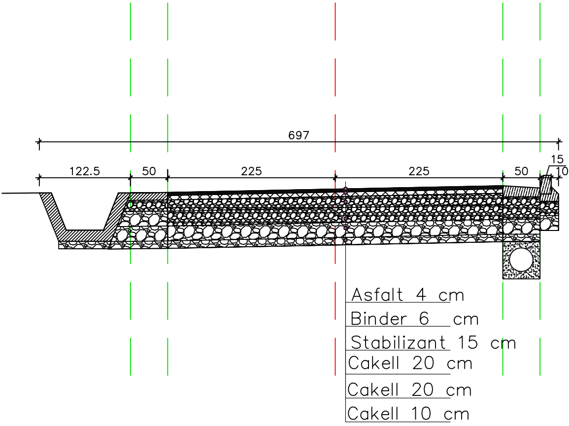
PROFIL TIP 2 Prog0+45.00-0+176.07
