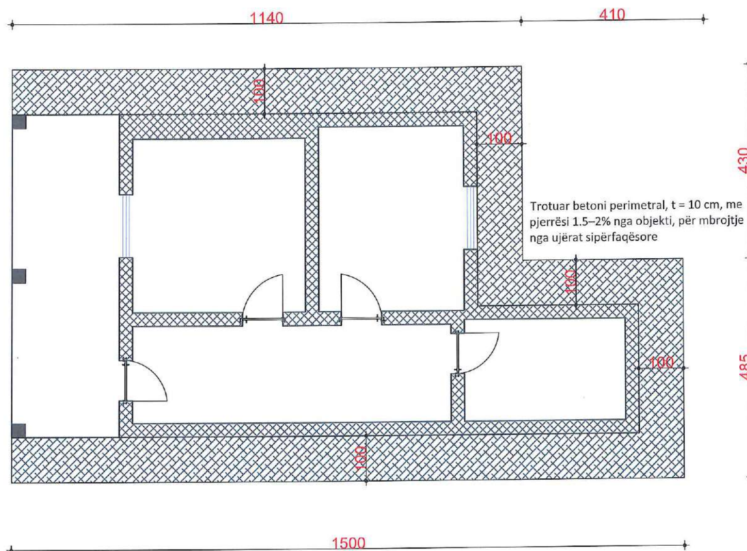
Planimetria e Katit Përdhe Sistemimi Perimetral i Objektit
