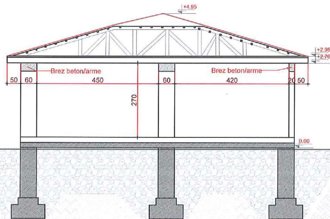
Fasada e Objektit
