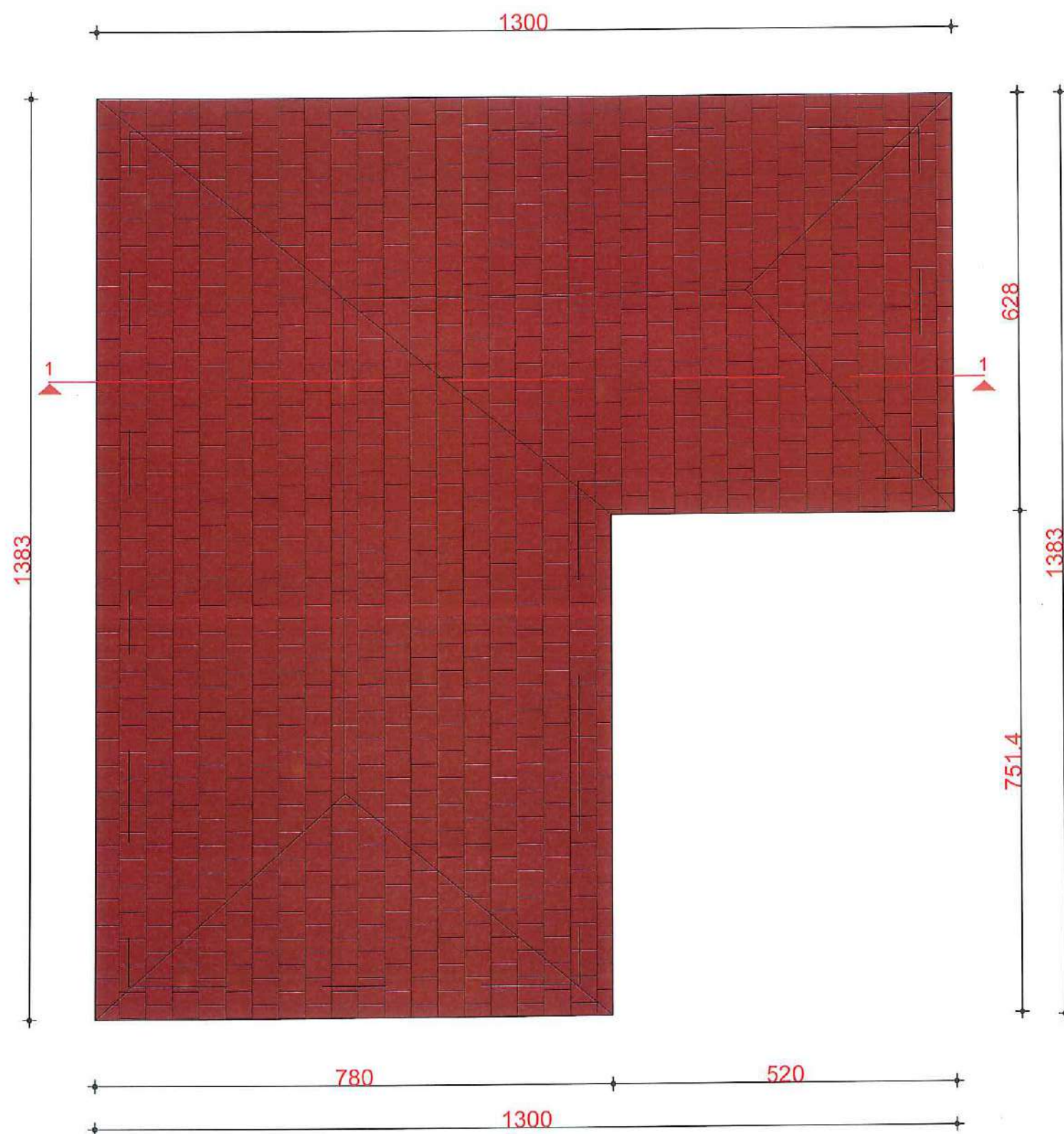
Planimetria e Çatisë
