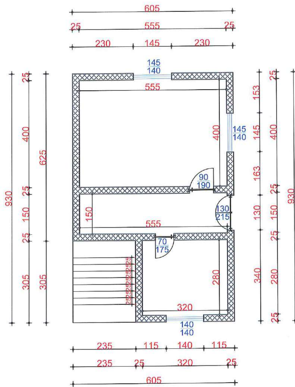
Planimetria e Katit Përdhe Kuota 0.00
