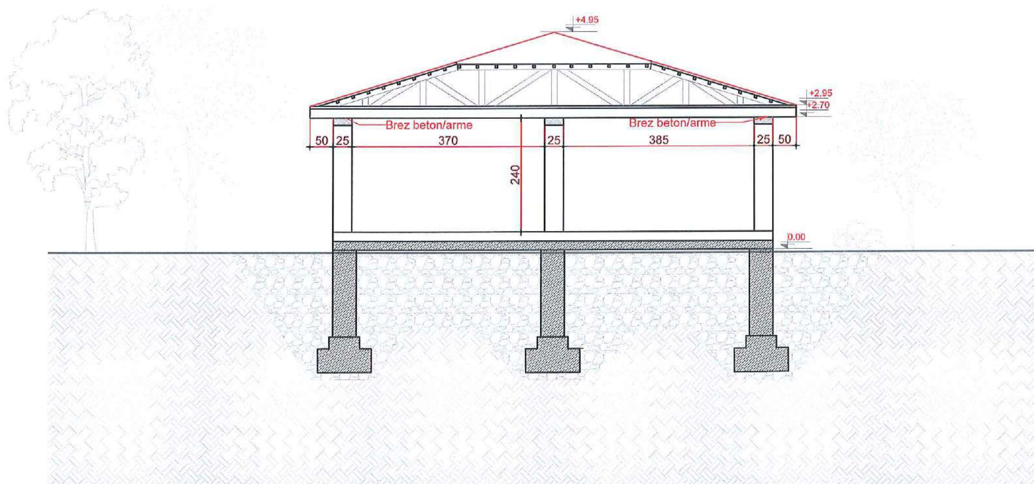
Fasada e Objektit
