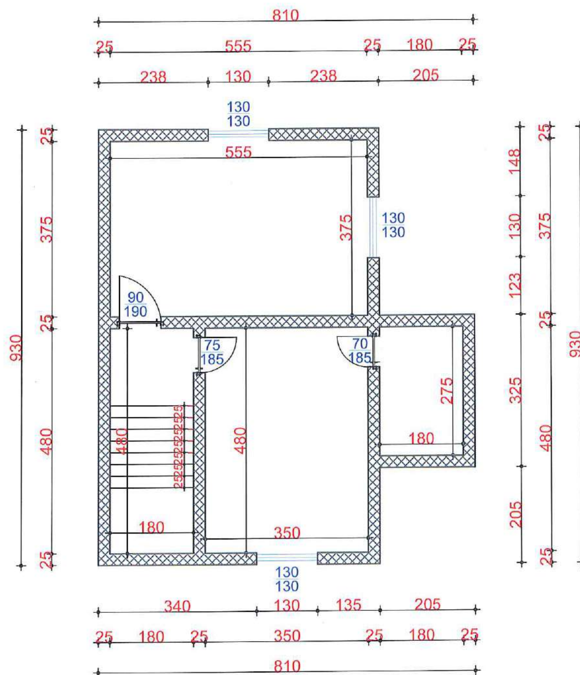
Planimetria e Katit të Parë Kuota +2.85
