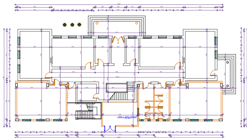
PLANIMETRIA E KATIT PERDHE Shk.1 :150
