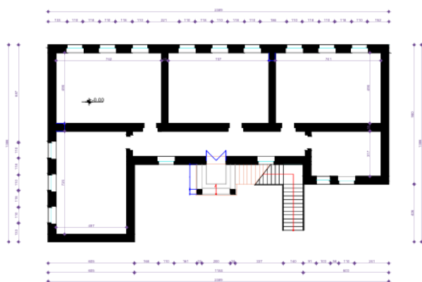
Plani i Katit Perdhe 0.00 SHKOLLA "NIKE LULI" KAMICE
