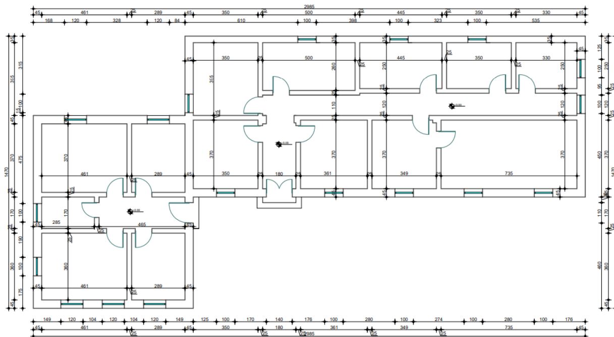
PLAN I KATIT PERDHE NJESIA ADMINISTRATIVE GRUEMIRE , MALES E MADHE SHK 1:100
