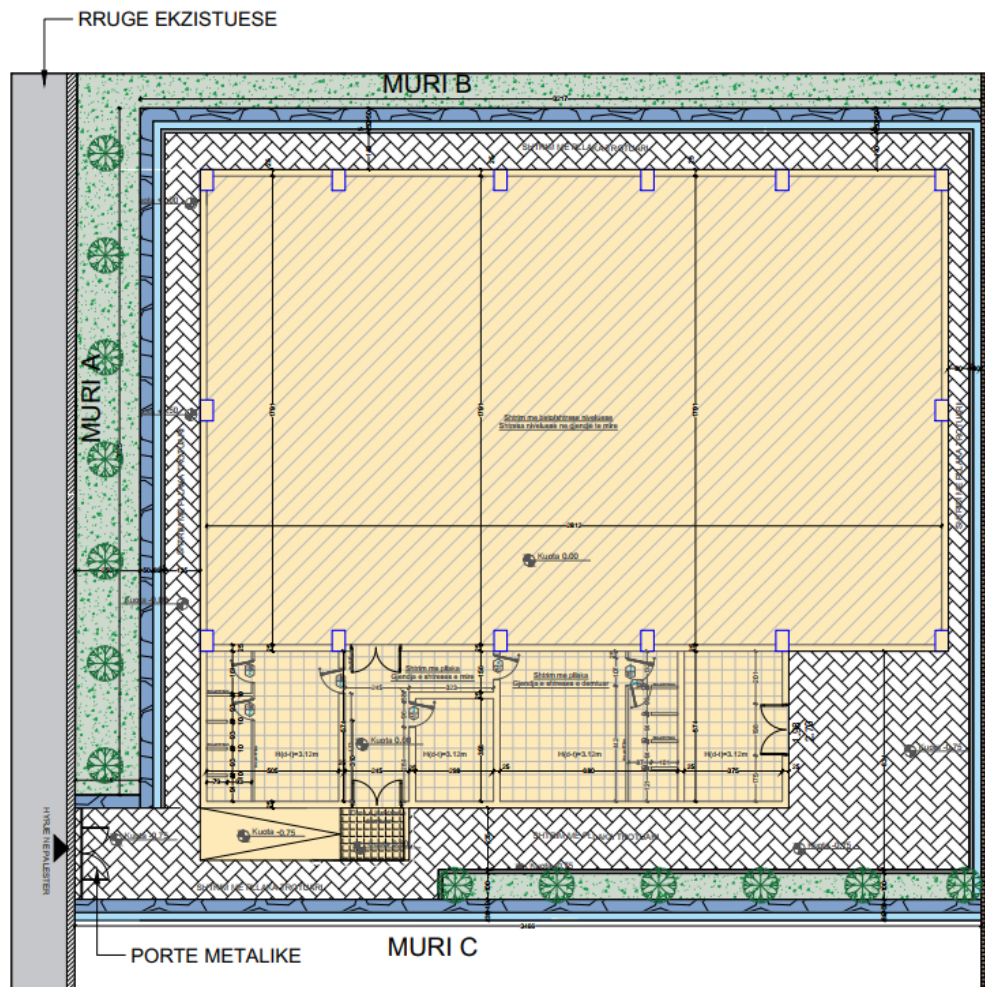
Fig.3. Plani i sistemimit i propozuar
