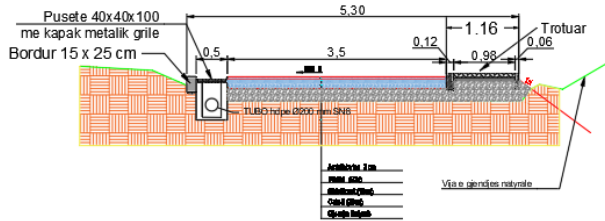
PROFILI TERTHOR 1 (DEGEZIMI) (0.00 m - 52,6 m dhe 59,6 m - 95 m ne degezim),NE AKSIN E PUSETES. SH 1: 50
