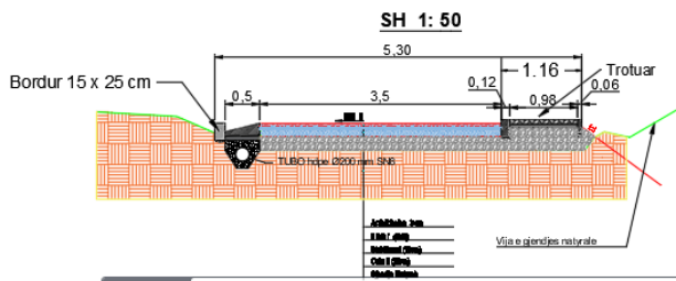
PROFILI TERTHOR 3 (DEGEZIMI) (0.00 m - 52,6 m dhe 59,6 m - 95 m ne degezim) JO NE AKSIN E PUSETES SH 1: 50
