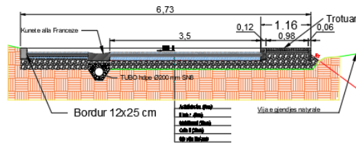
PROFILI TERTHOR 2 ( DEGEZIMI) (52,6 m - 59,6 m ne degezim) SH 1: 50
