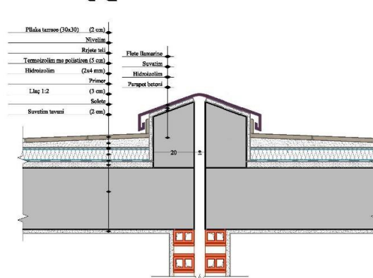
Detaj i fuges "F-2"
