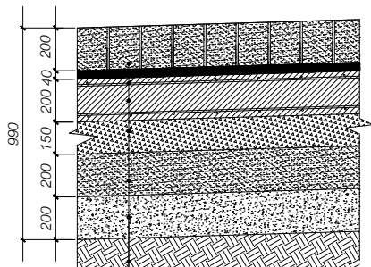
SEKSIONI 1-1 (prerja 7-9) Rifinitura: Plaka guri
