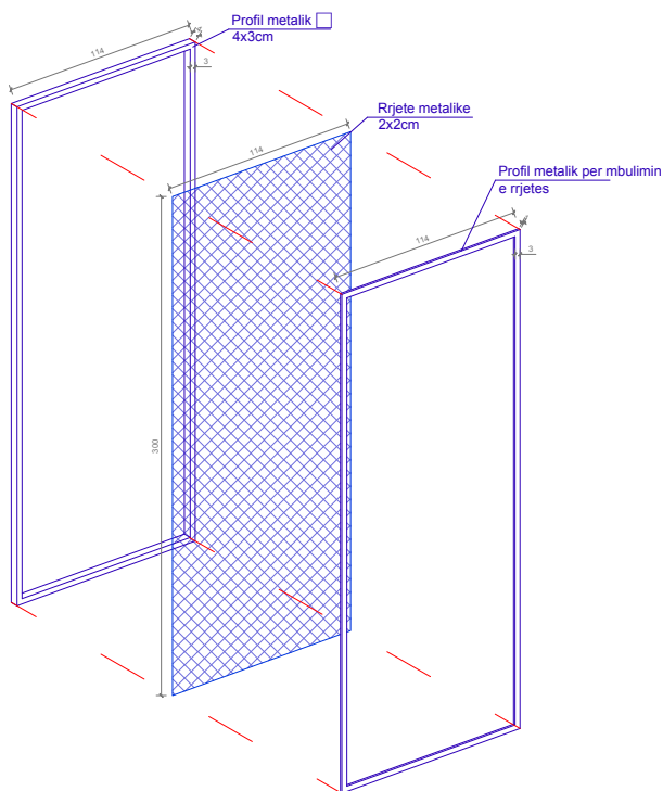
Aksonometri e panelit
