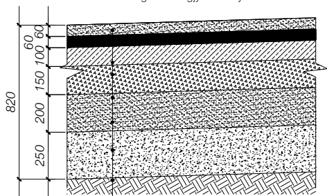
SEKSIONI 3-3 (prerja 22-25) Rifinitura: Asfalt me gure me ngjyra te ndryshme i rashinuar.
