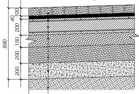
SEKSIONI 5 - 5 (prerja 32-36) Rifinitura: Plaka betoni speciale.
