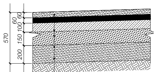
SEKSIONI 4-4 (prerja 4-6, 10-14, 16-21, 26-31, 37-43) Rifinitura: Asfalt me gure kuarci te shperndare.
