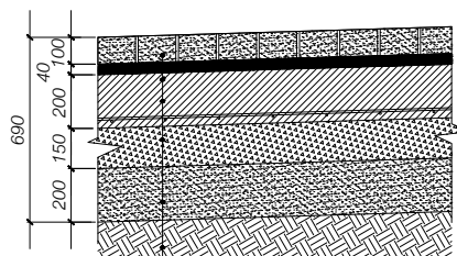
SEKSIONI 2-2 (prerja 7-9) Rifinitura: Plaka guri Shtresat ne zonat e destinuar per kembesore.
