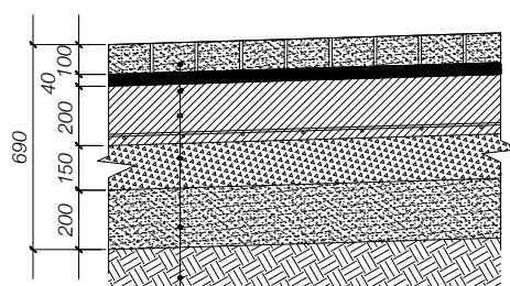
SEKSIONI 6 - 6 (prerja 32-36) Rifinitura: Plaka betoni speciale Shtresat ne zonat e destinuar per kembesore.
